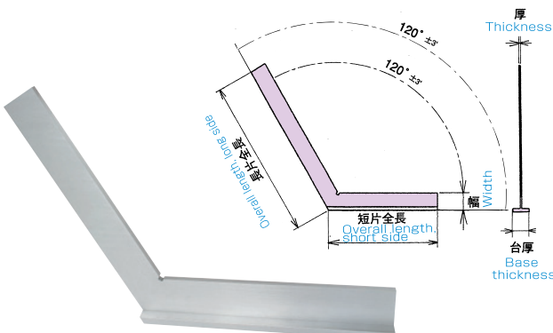
●OS-156E 寸法表 Dimensions OS-156E
