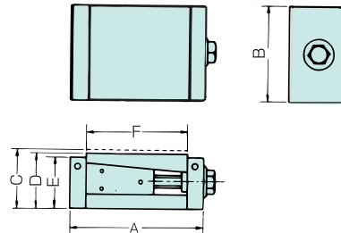
●OS-20T・30T・60T型 寸法表 Dimensions OS-20T・30T・60T type
