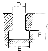
●T溝寸法図
