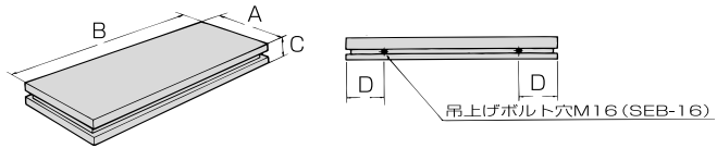
●プレート側面図
